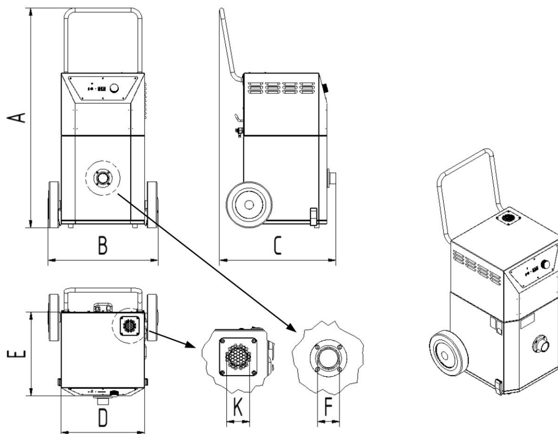
Obr. 15: Rozměrový výkres
