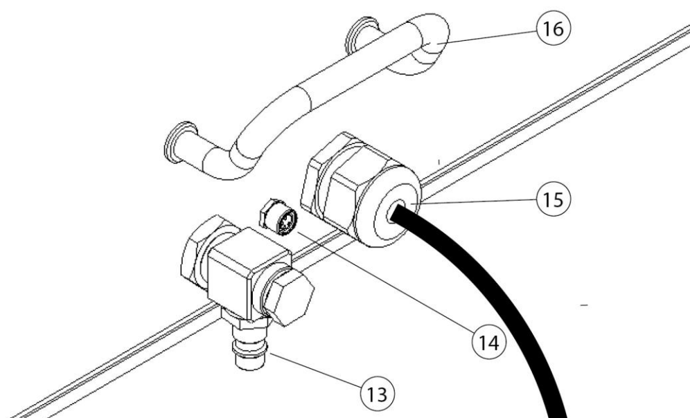
Obr. 2: Připojky
